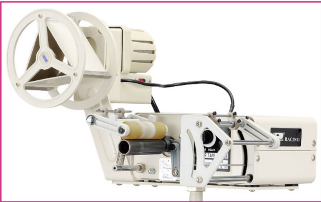
TFU 16-3 / UT-2 上送型送料機(附電動型防止打結裝置)，送料寬度70mm Upper tape feeder (with untangling motor device). Feed width 70mm TFU 16-8 上送型送料機，送料寬度 200mm Upper tape feeder, Feed width 200mm
